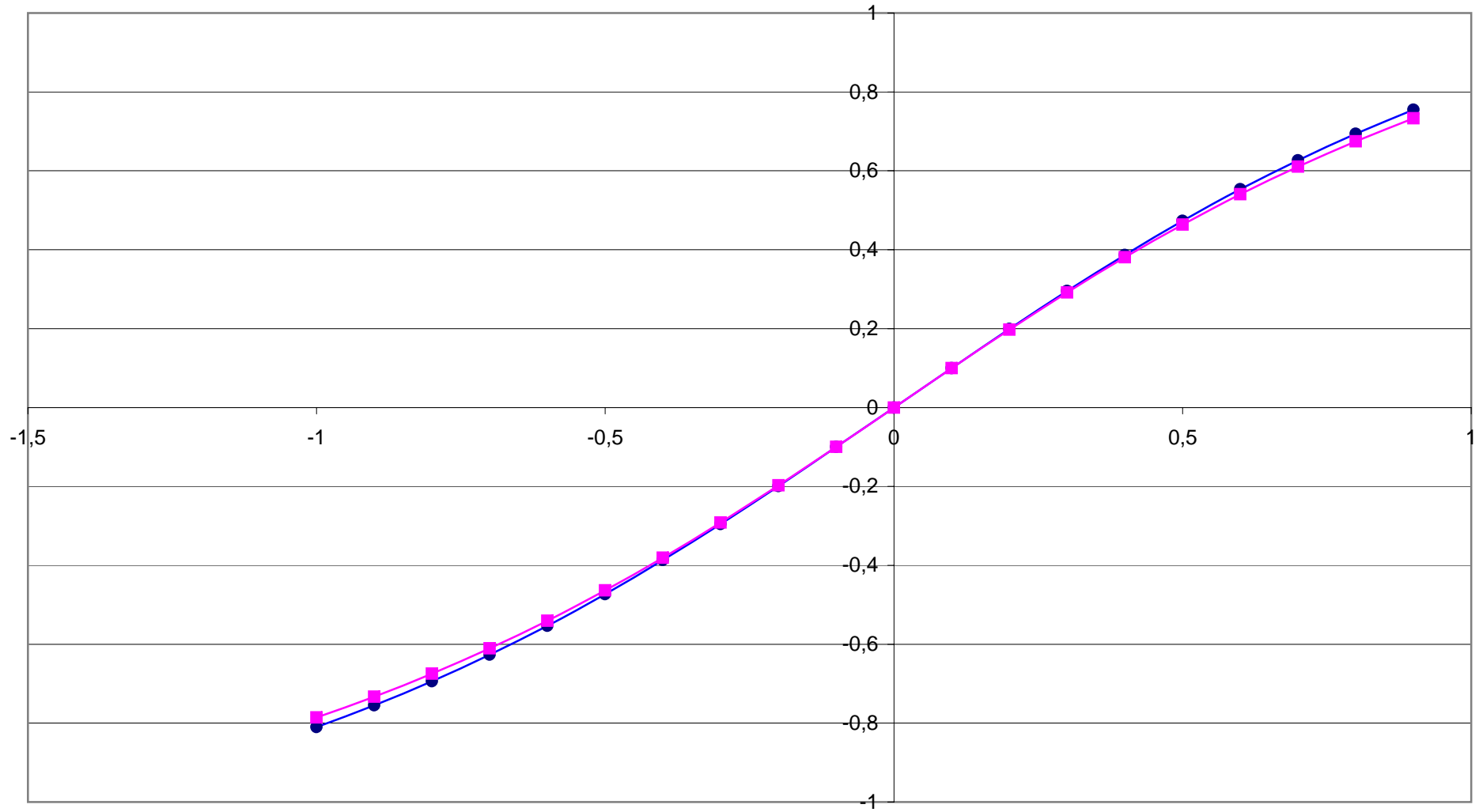
Méthode d'Euler , en bleue, la fonction exacte, en rose , l'approximation obtenue ( pas de 0,1)
